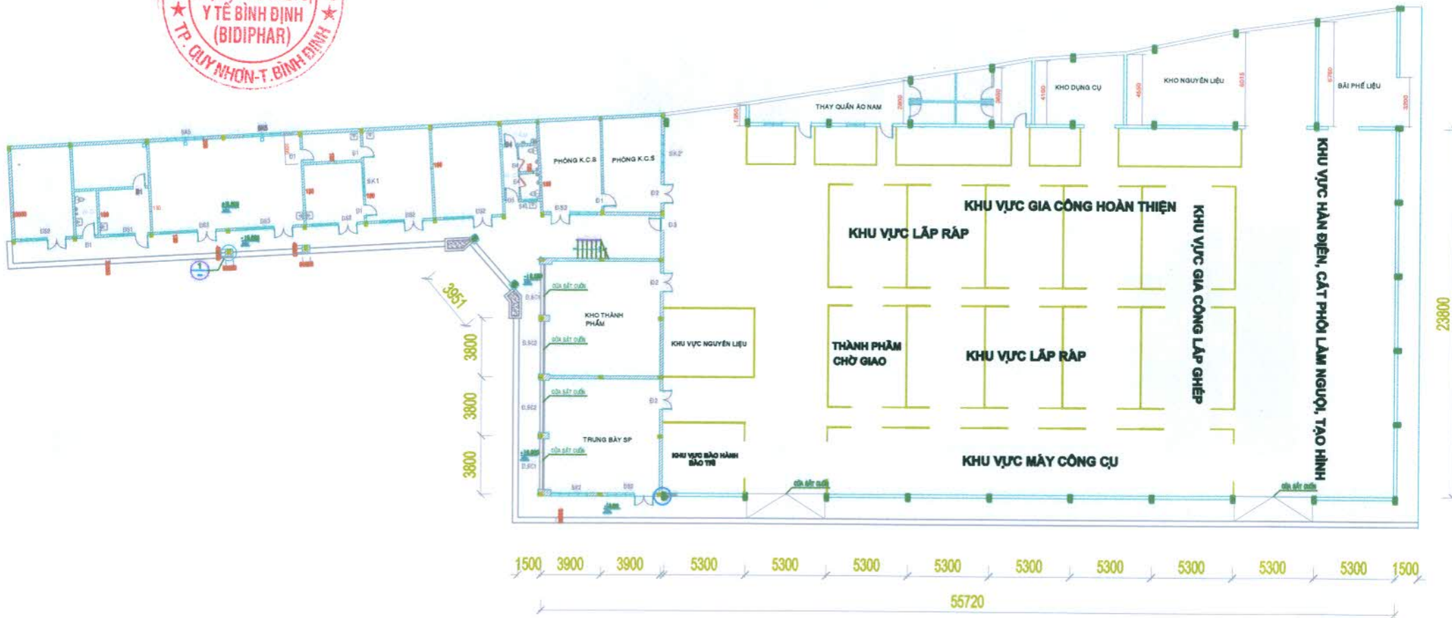
MẶT BẰNG HIỆN TRẠNG TẦNG 1
