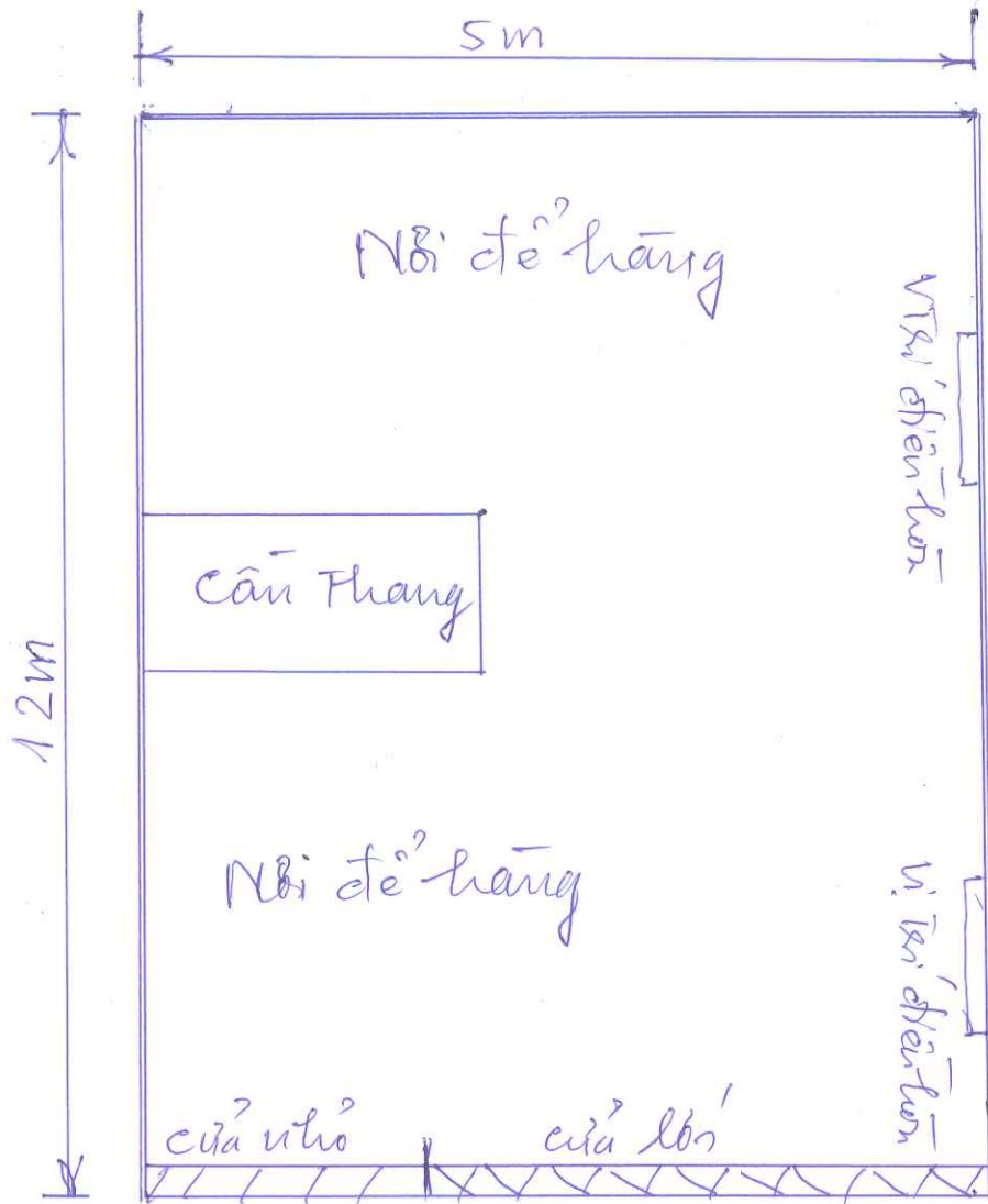
Mặt bằng T 1
