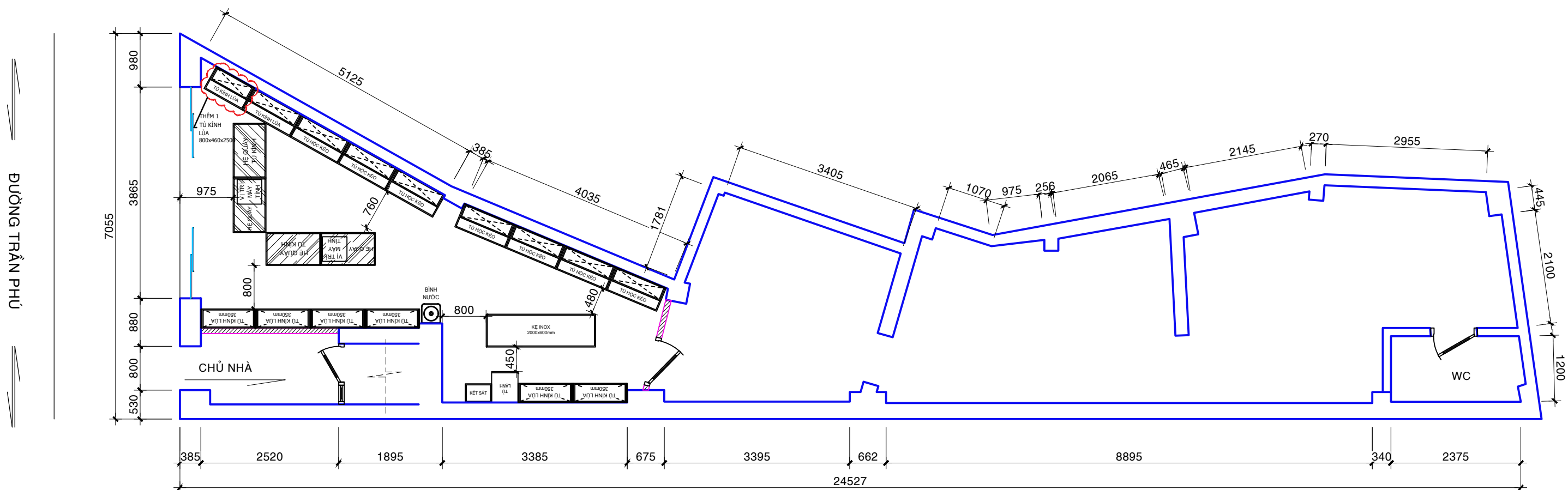
MẶT BẰNG BỐ TRÍ NỘI THẤT DIỆN TÍCH: 28m 2 TL: 1/75
