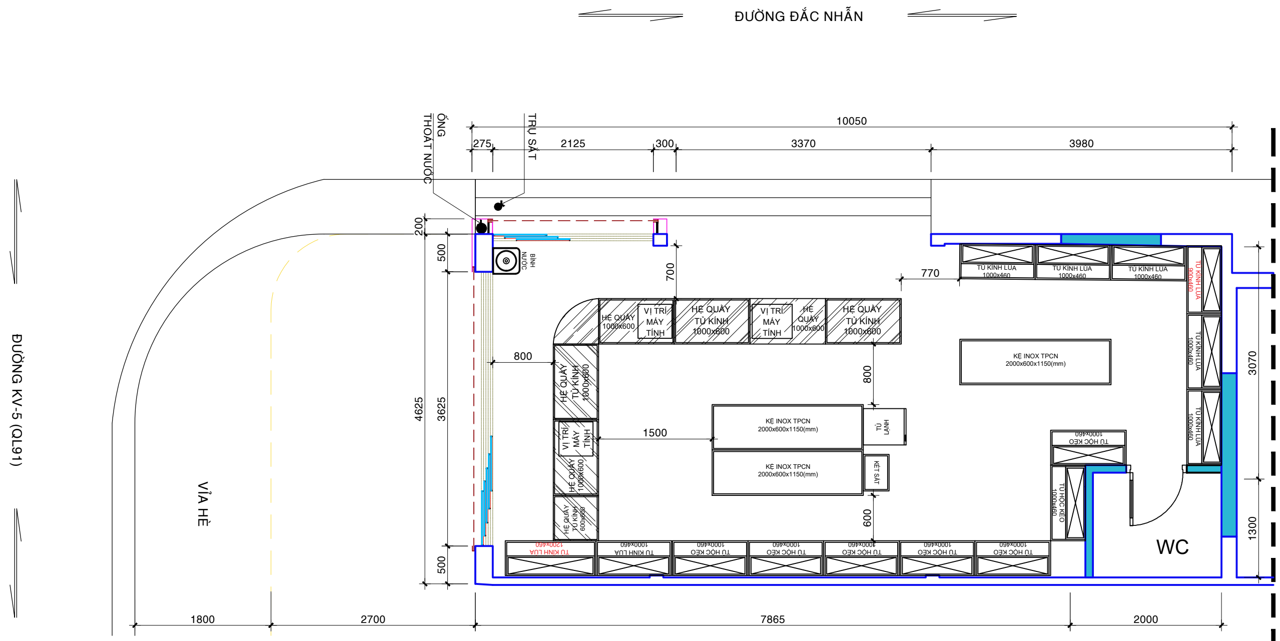
MẶT BẰNG BỐ TRÍ DIỆN TÍCH KINH DOANH: 40m 2 TL: 1/50
