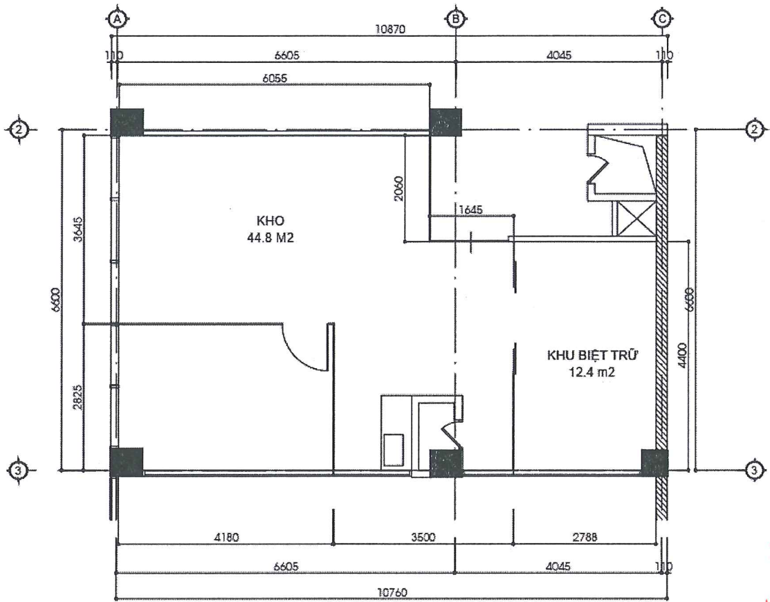
Hình 1: Sơ đồ bố trí kho bảo quản trang thiết bị y tế của Công ty CP Đầu tư Công nghệ HP Việt Nam
