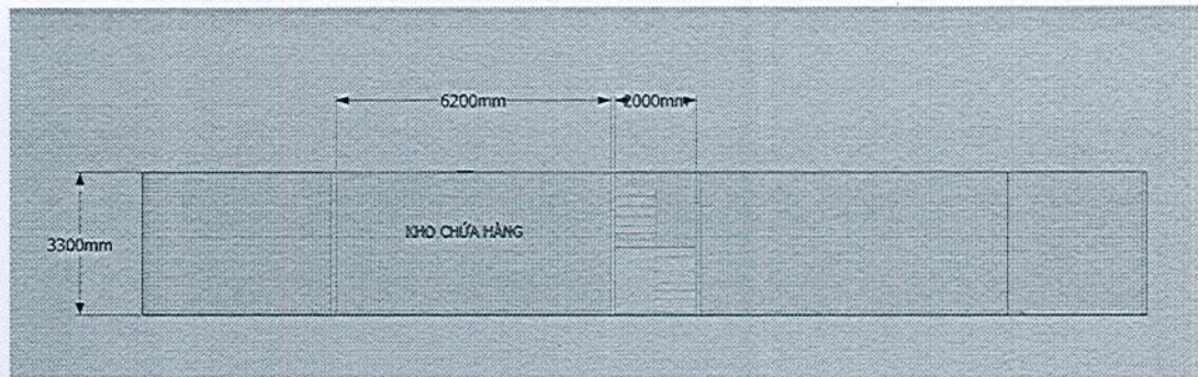
MAT CẮT DỌC
